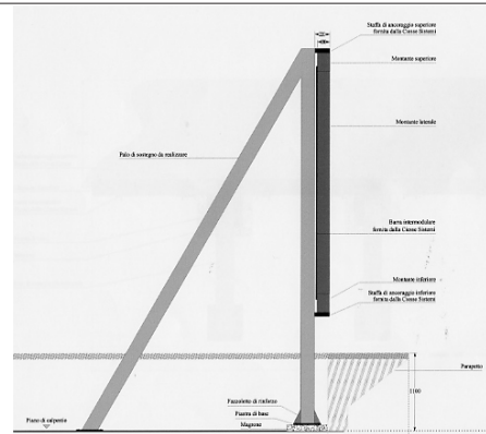
Prospetto retro
